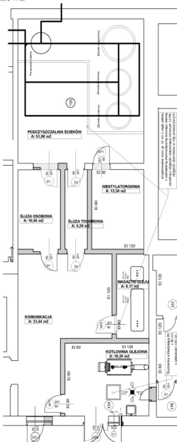
SZKIC IDEOWY UKŁADU PRZEBUDOWYWANYCH POMIESZCZEŃ
